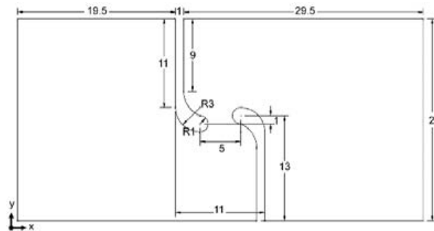
Figura 2 – Probeta para ensayo de cortante puro con sus respectivas dimensiones en milímetros.
