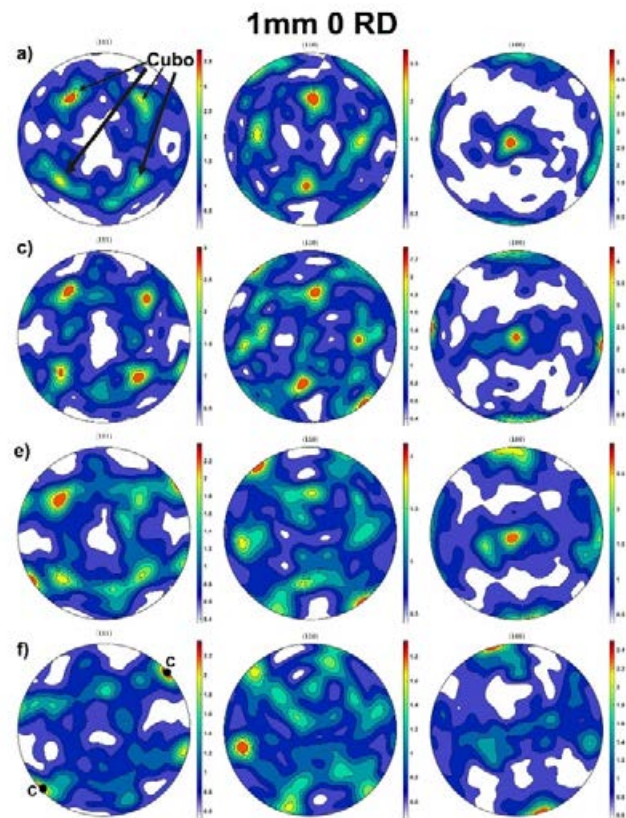
Figura 11 – Figuras de polo correspondientes a la probeta 1 mm 0 RD a 1.25 mm de desplazamiento. Las figuras a) fueron medidas lejos de la zona cortante, mientras que las figuras f) se midieron directamente en la zona cortante.
