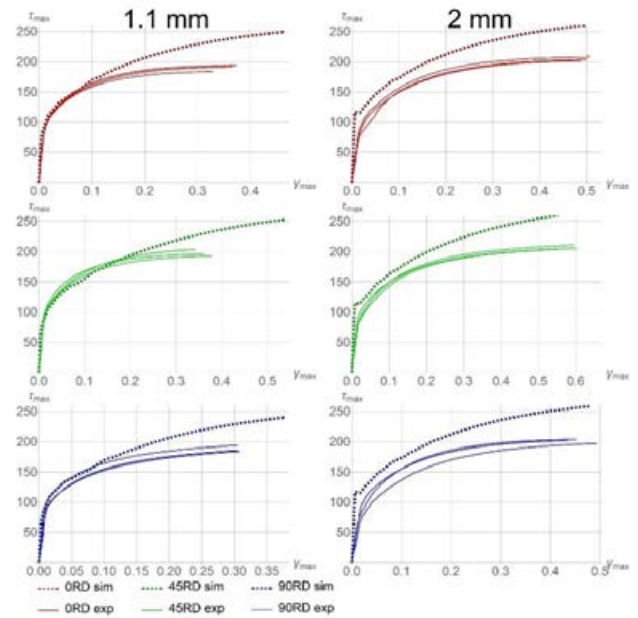
Figura 8– Curvas de deformación cortante máxima vs esfuerzo cortante máximo en los distintos ensayos (líneas sólidas) con sus respectivas simulaciones (líneas punteadas).
