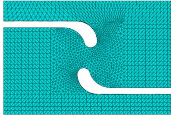
Figura 4 – Mallado aplicado a la probeta.
