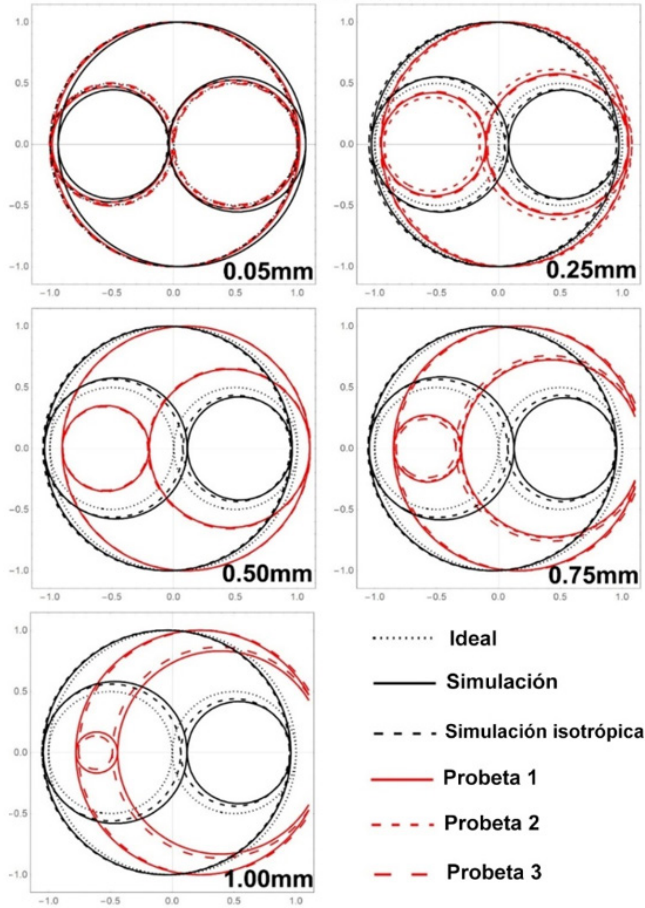
Figura 9 – Círculos de Mohr normalizados de las tres probetas ensayadas (líneas rojas), de simulación isotrópica (líneas negras con guiones) y anisotrópica mediante HMS (línea negra sólida) en varios desplazamientos para probeta de 1.1 mm 0RD
