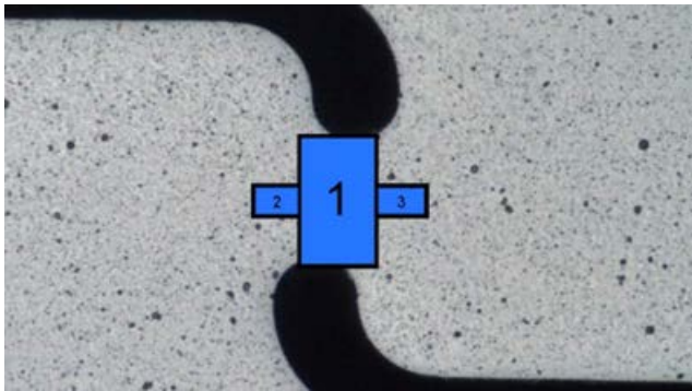
Figura 6– Zona de las probetas donde la textura fue medida.
