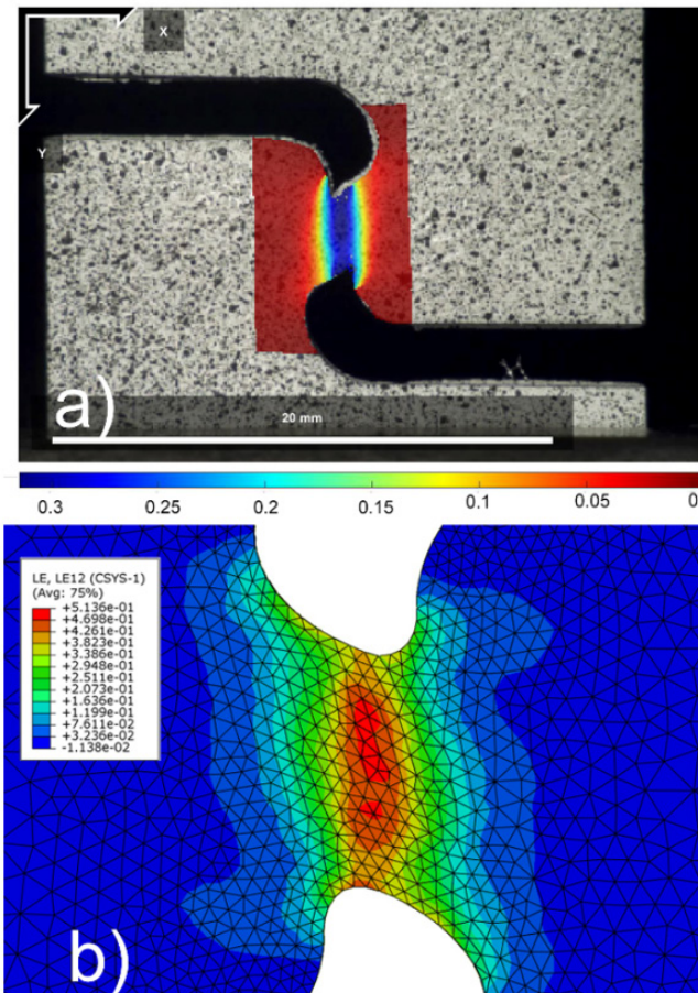
Figura 7– Componente de deformación cortante a 1.25 mm de desplazamiento para probeta de 1.1 mm de espesor en 0 RD en a) DIC y b) simulación con ley de endurecimiento de Voce.
