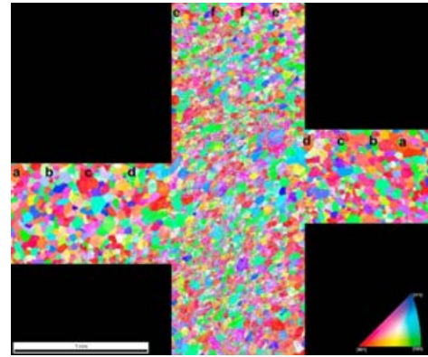
Figura 10 – IPFM de probeta 2 mm 0 RD parcialmente ensayada. Las letras muestran las secciones en que fue dividida la medición para obtener las distintas figuras de polo y ODFs.
