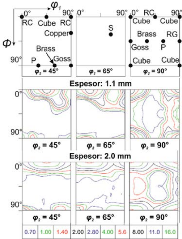
Figura 3 – Secciones ODF de la textura de la aleación 6016 en espesores de 1.1 y 2 mm. Se muestran las secciones de 0 a 90° y \phi_2 en 45°, 65° y 90° [11].
