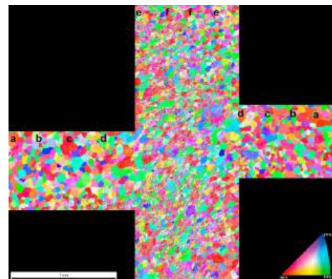
Figura 10 – IPFM de probeta 2 mm 0 RD parcialmente ensayada. Las letras muestran las secciones en que fue dividida la medición para obtener las distintas figuras de polo y ODFs.
