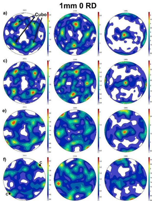
Figura 11 – Figuras de polo correspondientes a la probeta 1 mm 0 RD a 1.25 mm de desplazamiento. Las figuras a) fueron medidas lejos de la zona cortante, mientras que las figuras f) se midieron directamente en la zona cortante.
