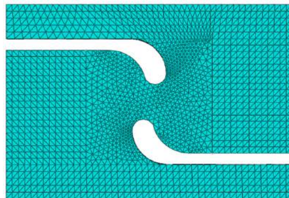
Figura 4 – Mallado aplicado a la probeta.
